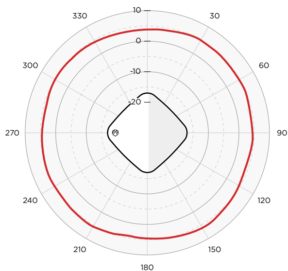
Azymut - 2.4 GHz
