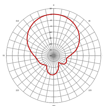
Vertical (ETSI)
